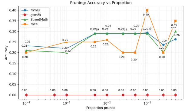
(d) Pruning accuracy on Dream-v0-Instruct-7B
